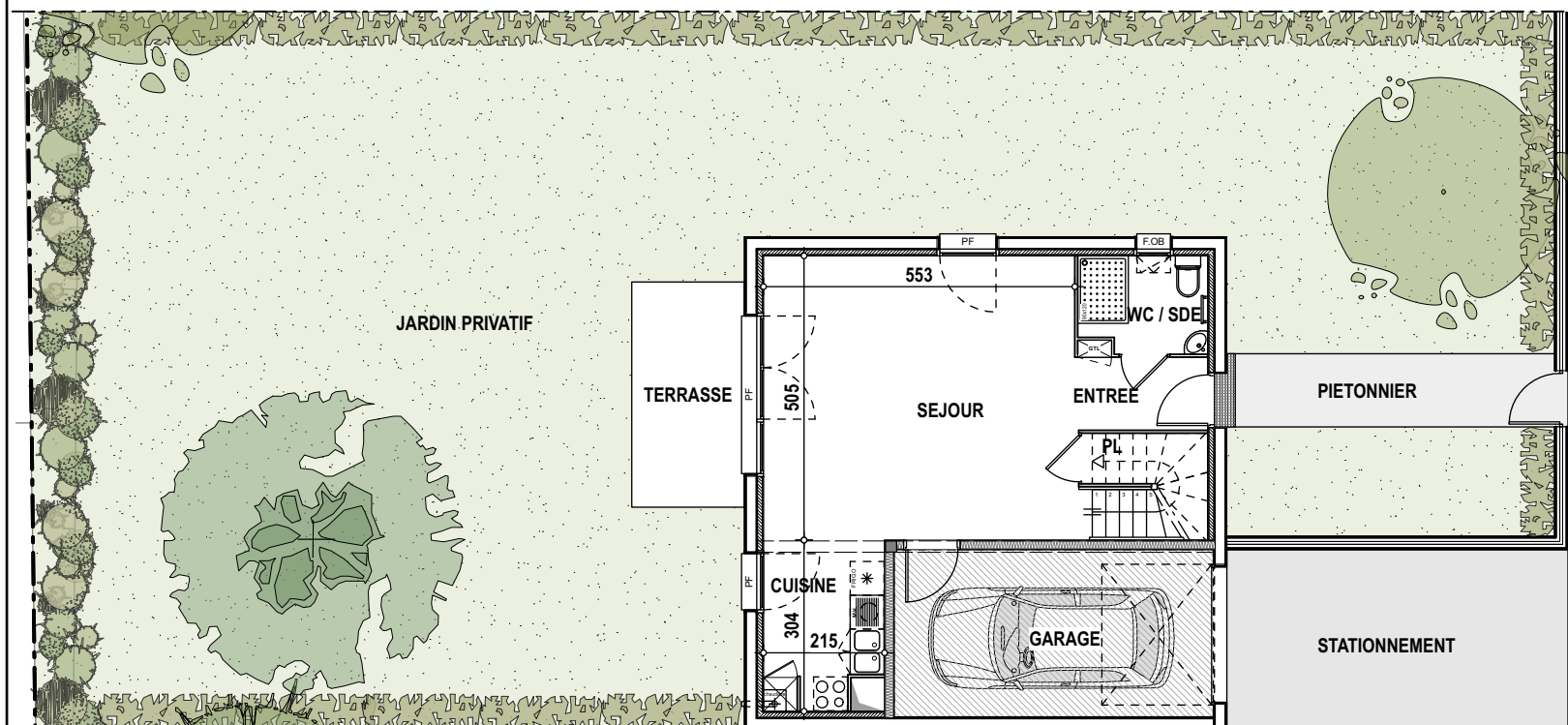
REZ-DE-CHAUSSEE
