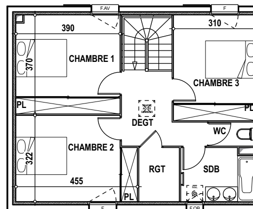
ETAGE
